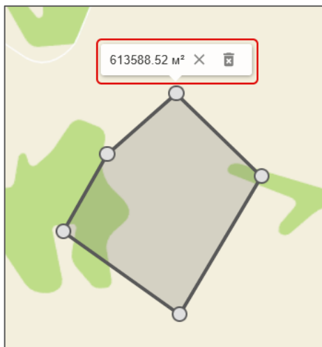
Рисунок 21 – Площадь
