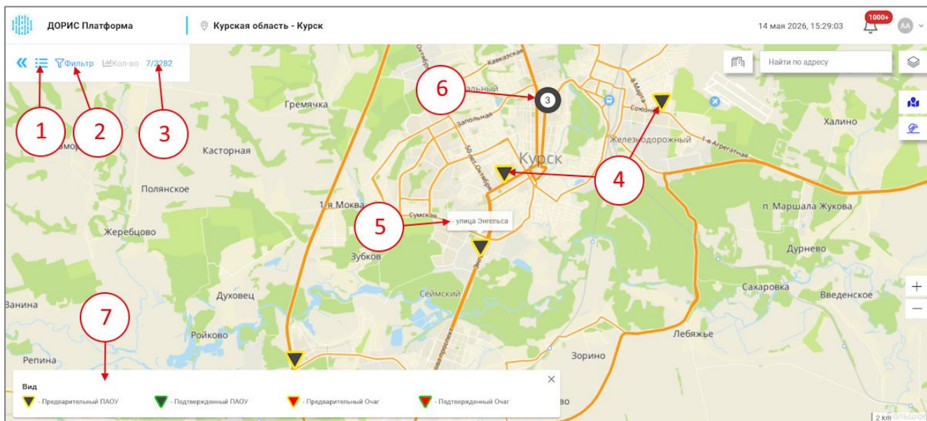
Рисунок 194 – Страница «МКДТП»
