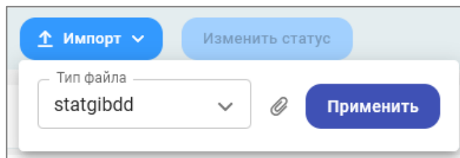
Рисунок 238 – Импорт
