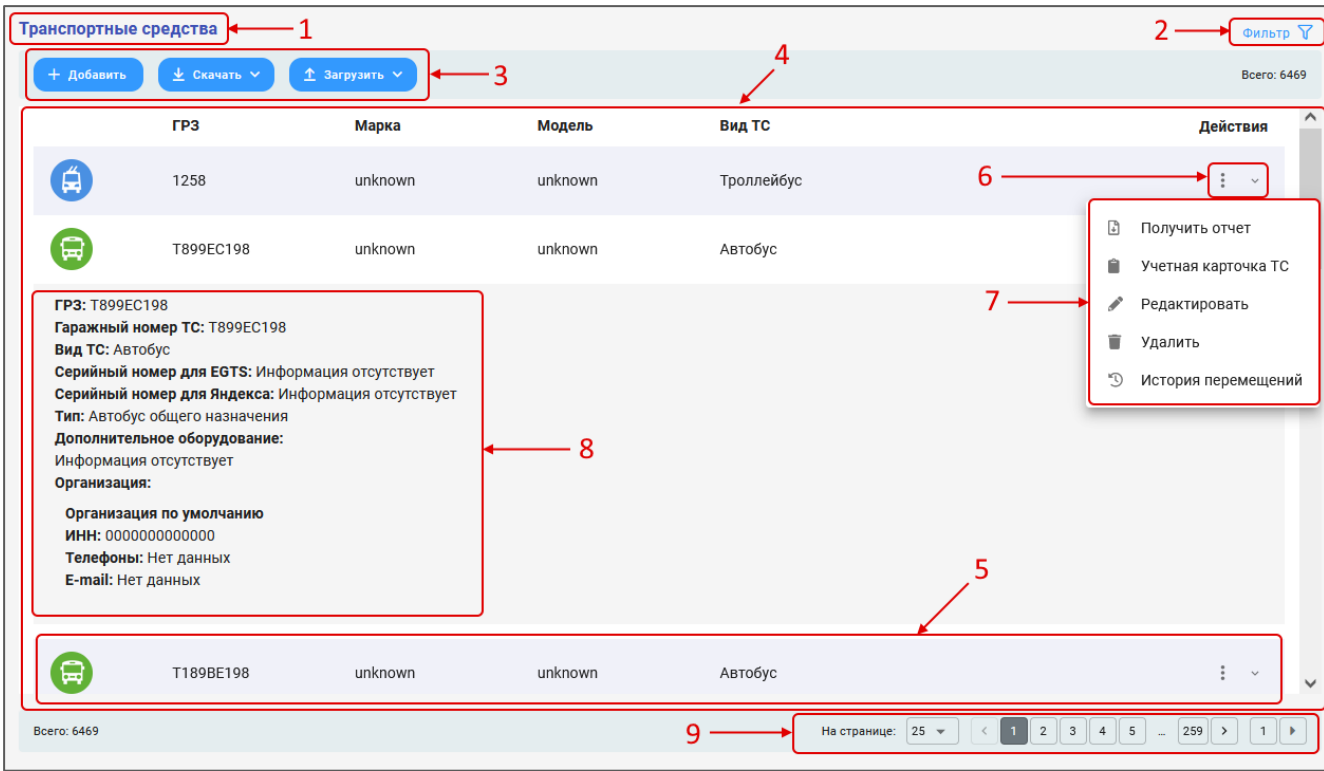
Рисунок 86 – Транспортные средства
