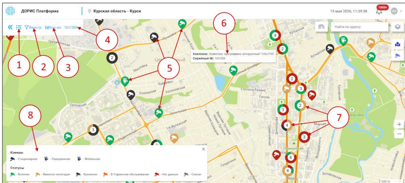
Рисунок 28 –«На карте»
