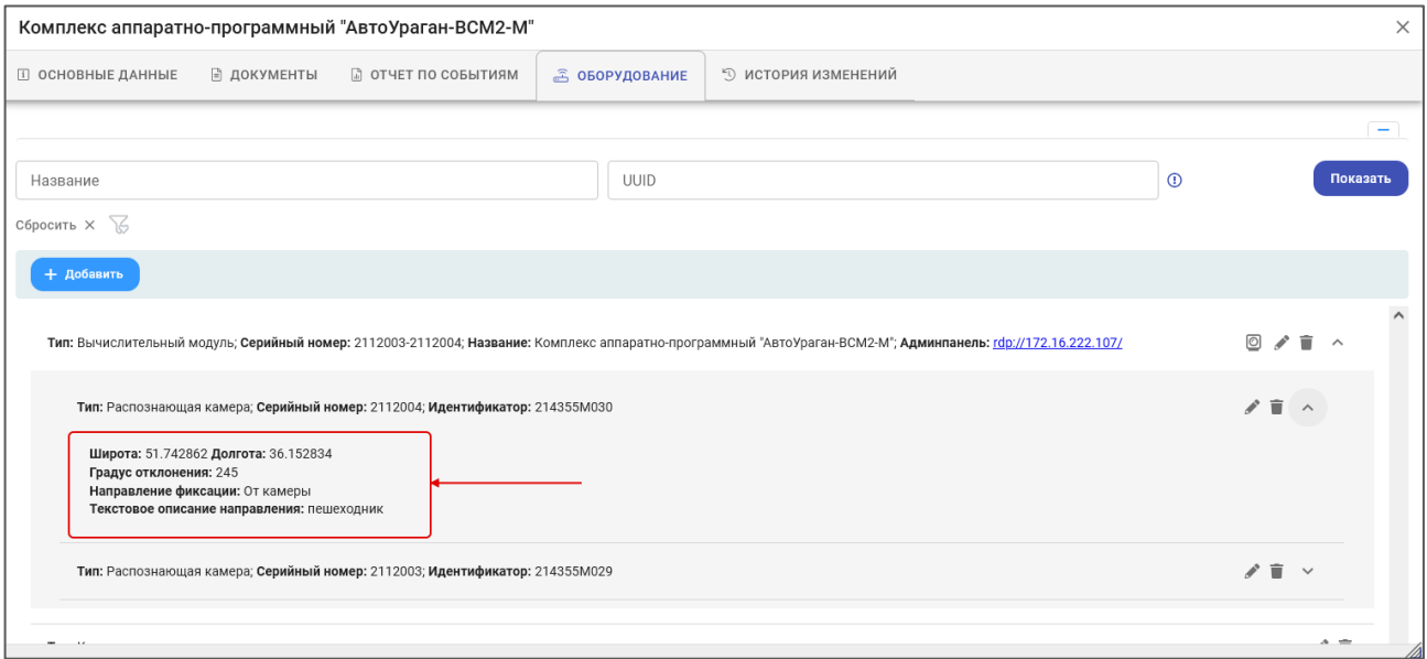
Рисунок 56 – Вкладка «Оборудование»
