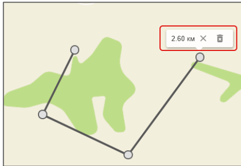
Рисунок 20 – Длина
