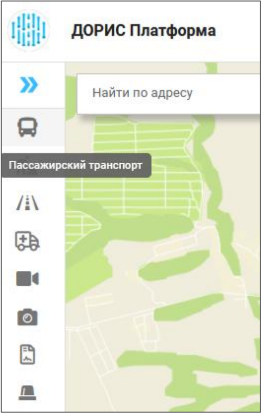
Рисунок 3. Свёрнутое меню
