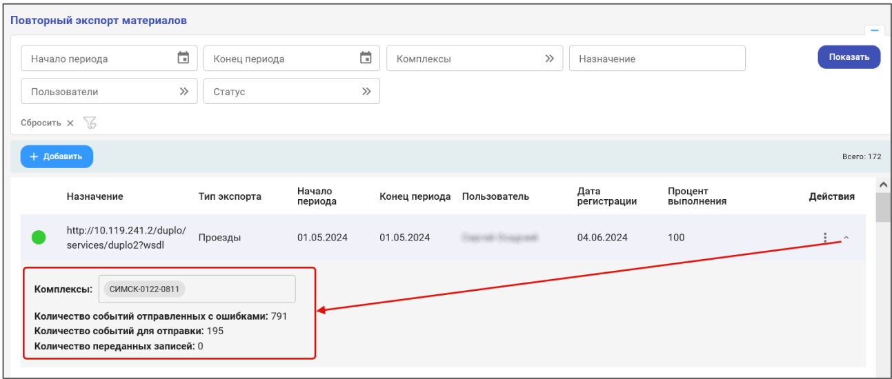
Рисунок 107 – Подробный просмотр
