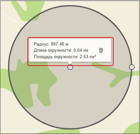
Рисунок 22 – Окружность
