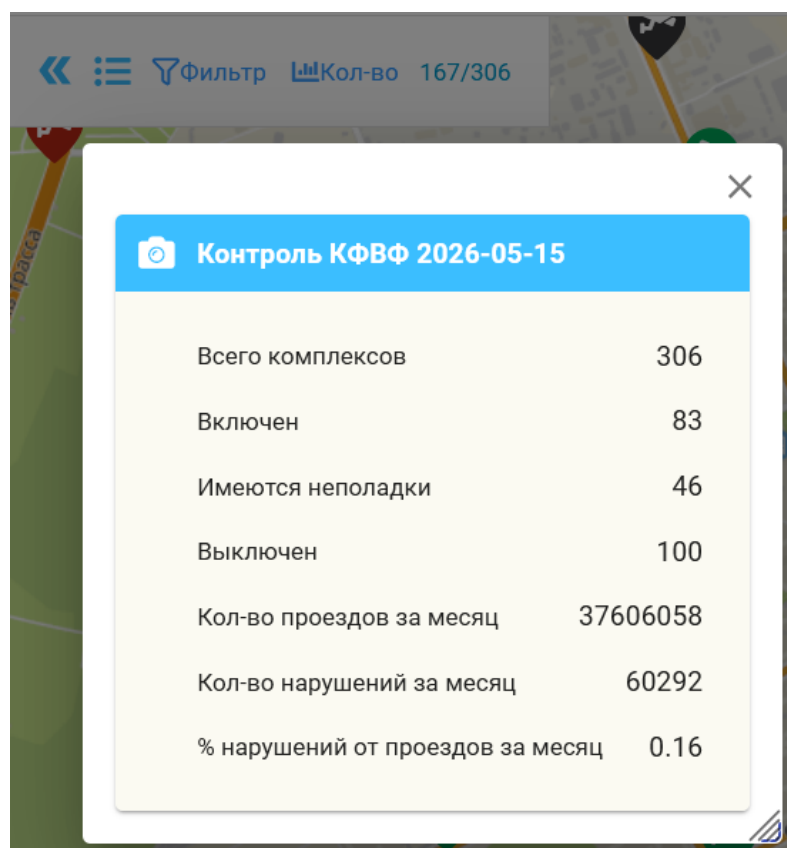
Рисунок 29 – Статистика
