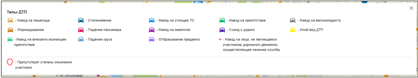
Рисунок 159. Легенда
