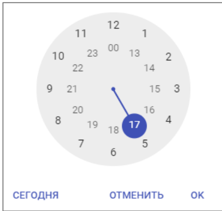
Рисунок 294 – Часы.
